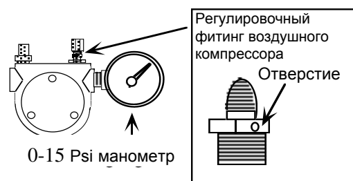
Расположение компрессора
