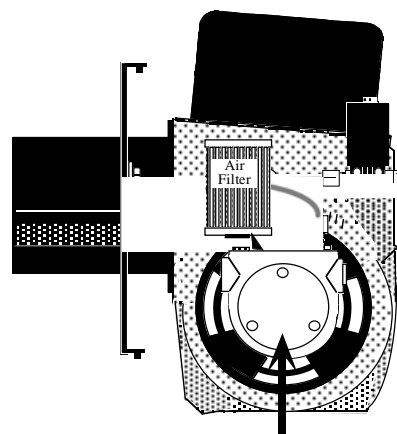
Расположение компрессора
